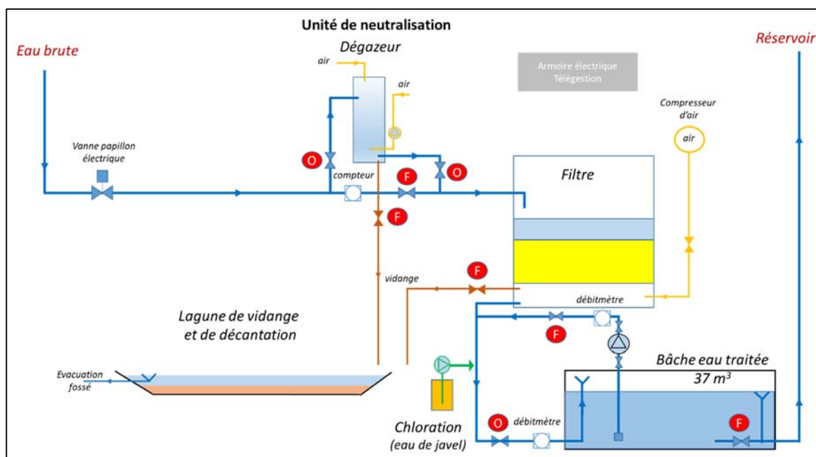
Figure 5 : exemple de schéma fonctionnel d'une unité de neutralisation (fiche complète en annexe)
