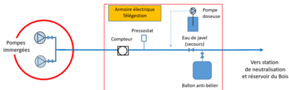
Figure 4 : exemple de fiche descriptive d'un captage (exemple de fiche complète en annexe)
