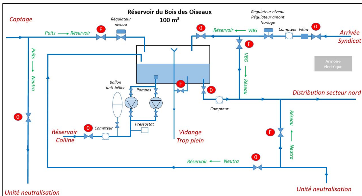
Figure 6 : exemple de schéma fonctionnel d'un réservoir
